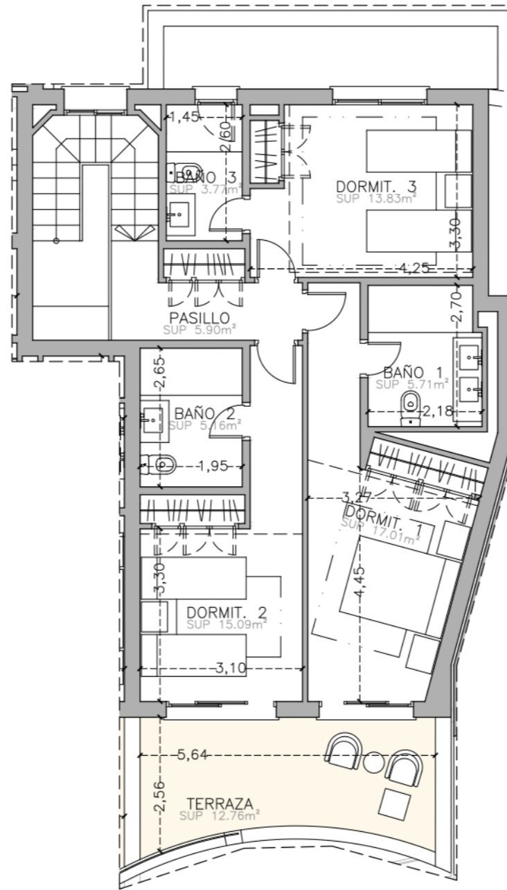
PLANTA PRIMERA
