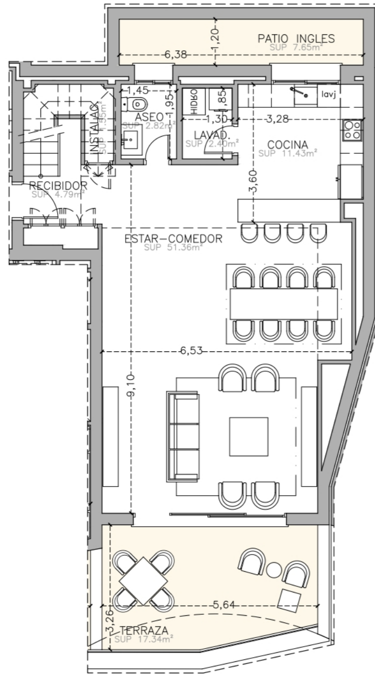
PLANTA 0
