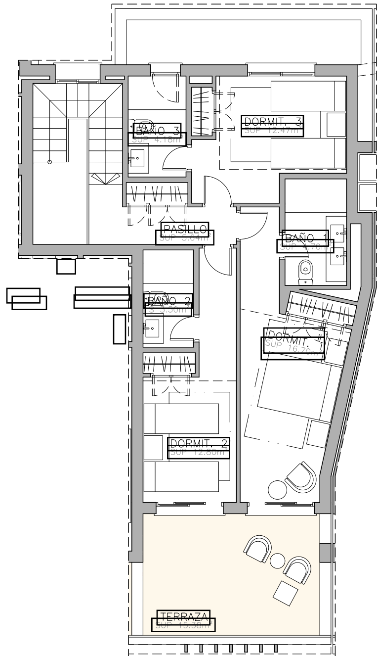
PLANTA PRIMERA
